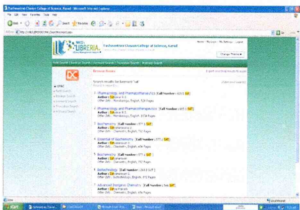
Web OPAC
